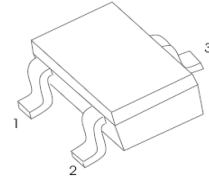
SOT-523
