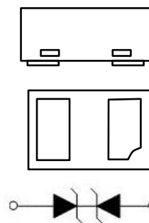
DFNWB1.0X0.6-02L
